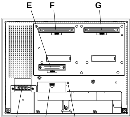
D H I 背部 (GP-2500/2600系列)
