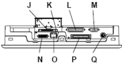
底部 (GP-2500/2600系列)
