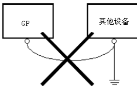
(c) 共用接地（不可行）
