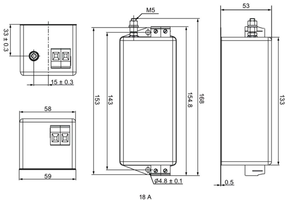
用于三相电网的滤波器
