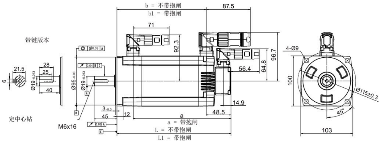
轴高 50 mm，带直角连接器
