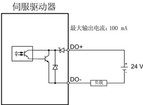
PNP 接线
