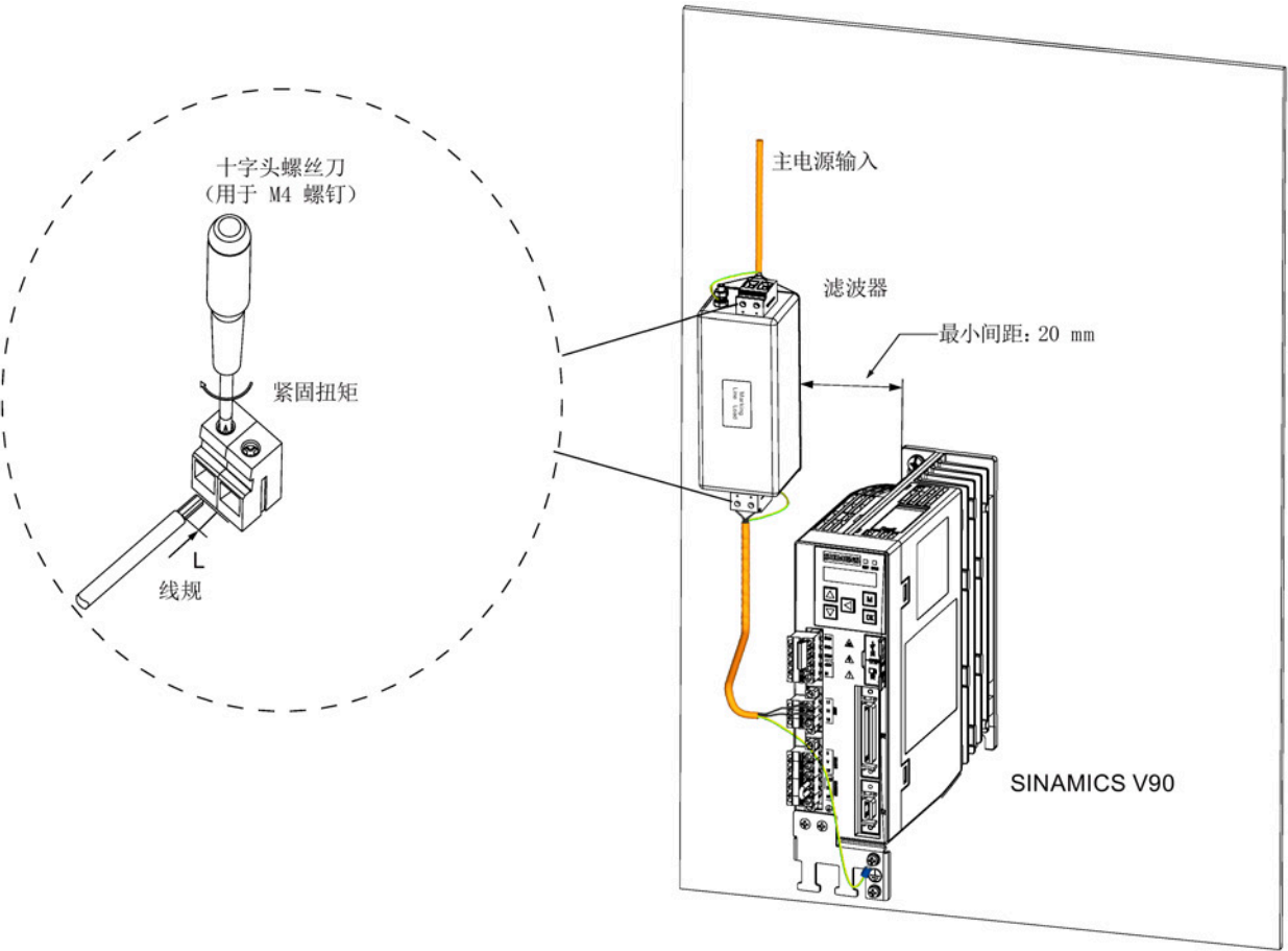
用于单相电网的滤波器
