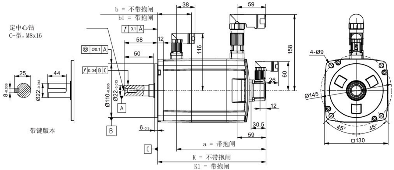
轴高 65 mm，带绝对值编码器和直角连接器
