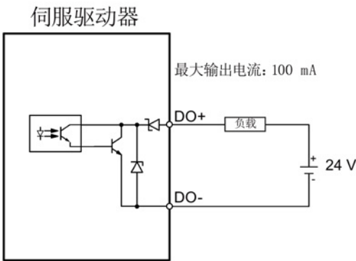
NPN 接线
