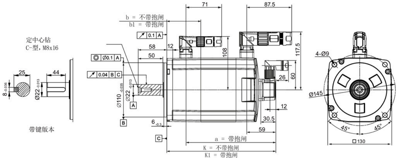
轴高 65 mm，带绝对值编码器和直角连接器
