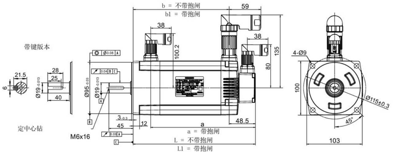
轴高 50 mm，带直角连接器
