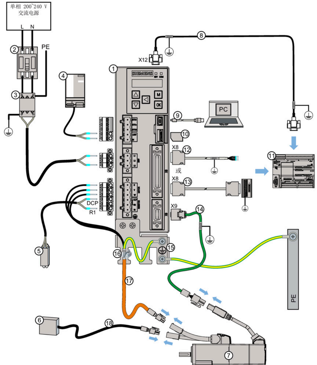
FSB 用于单相电网的连接图
