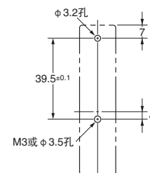
安装孔加工尺寸
