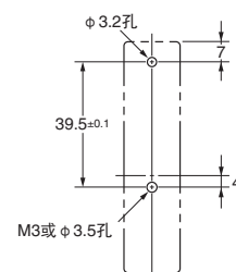
安装孔加工尺寸
