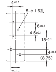
安装孔加工尺寸 (底视图)
