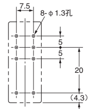
安装孔加工尺寸 (底视图)
