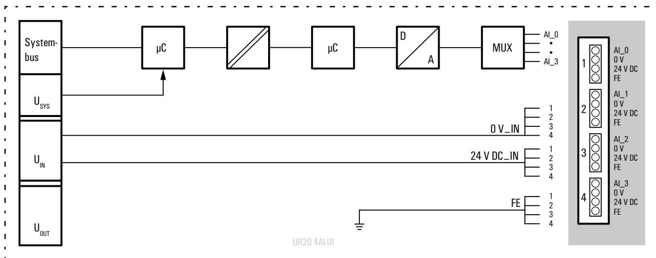
电路框图：UR20-4AI-UI-16
