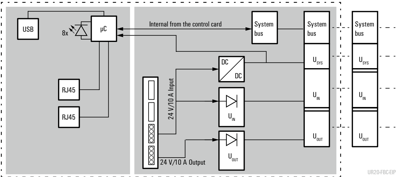
电路框图：UR20-FBC-MOD-EIP
