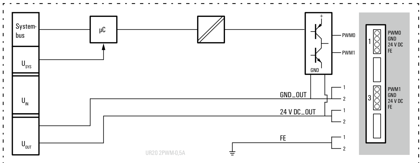
电路框图：UR20-2PWM-0.5 A
