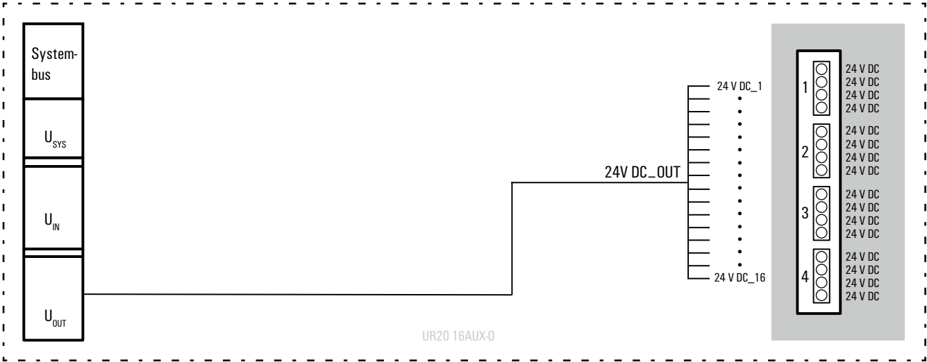
电路框图：UR20-16AUX-O
