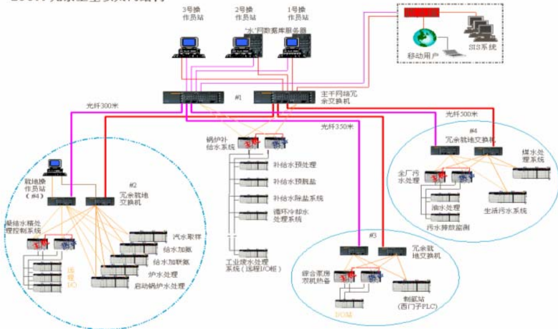
‘水’网集中监控系统网络结构图
