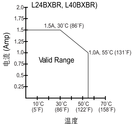
场效应晶体管 每点电流 (1762-L24BXB, L40BXB, L24BXBR, L40BXBR)
